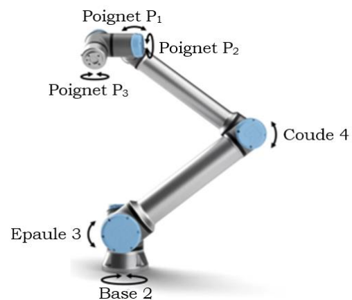
Figure 2 : Manipulateur Ur
