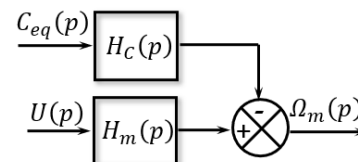
Figure 8 : Schéma équivalent du moteur
