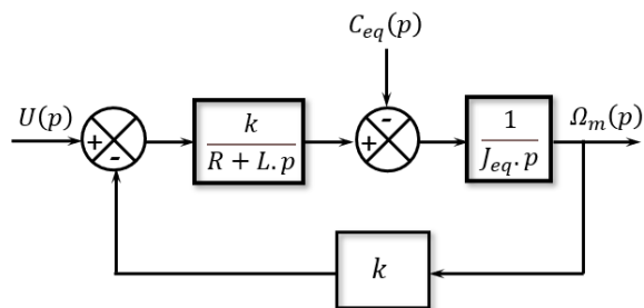
Figure 7 : Schéma blocs du moteur
