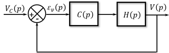
Figure 9 : Schéma bloc à retour unitaire
