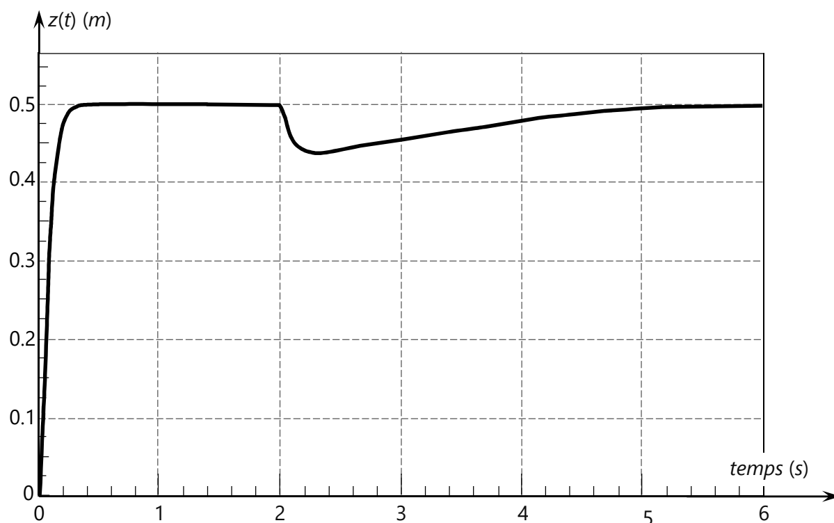
Figure R3 : Réponse du système à une consigne z_c(t) = 0,5.h(t) et une perturbation C_r(t) = 1,2.h(t - 2)
