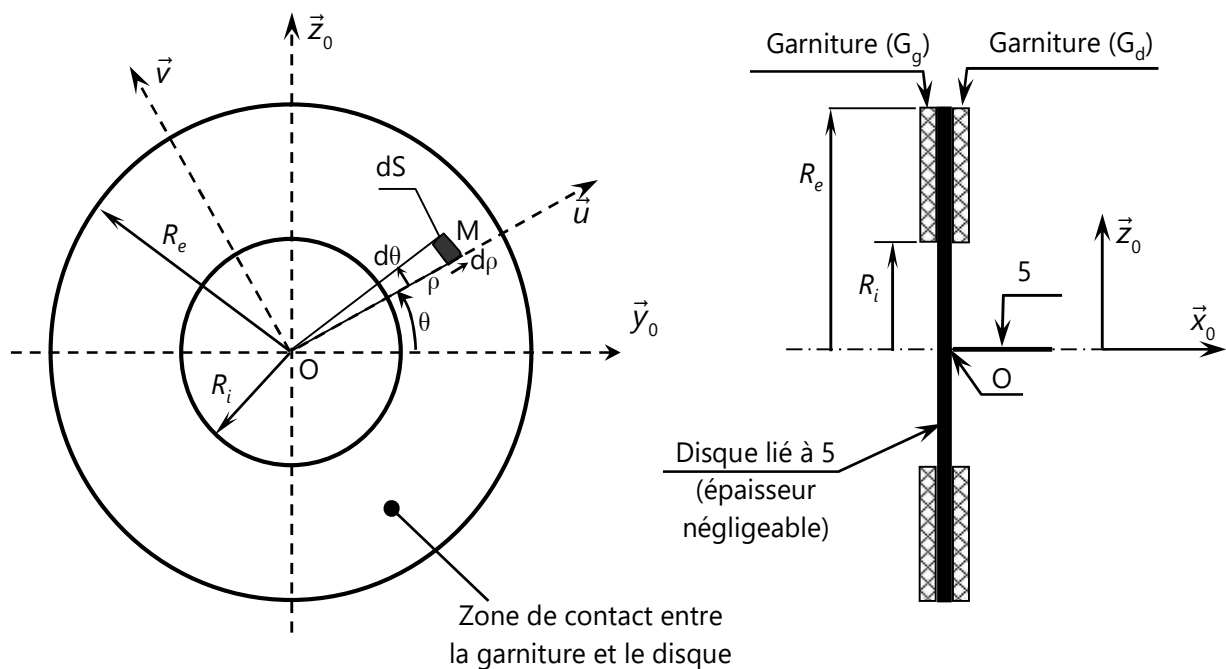
Figure 6 : Modèle retenu pour le frein
