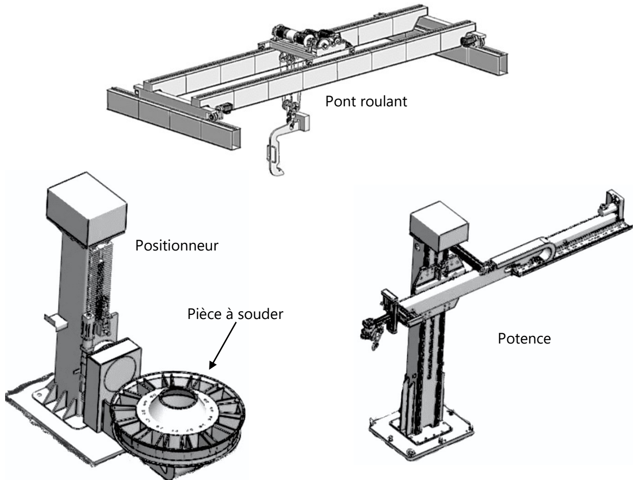
Figure 1 : Poste de soudage automatisé.
