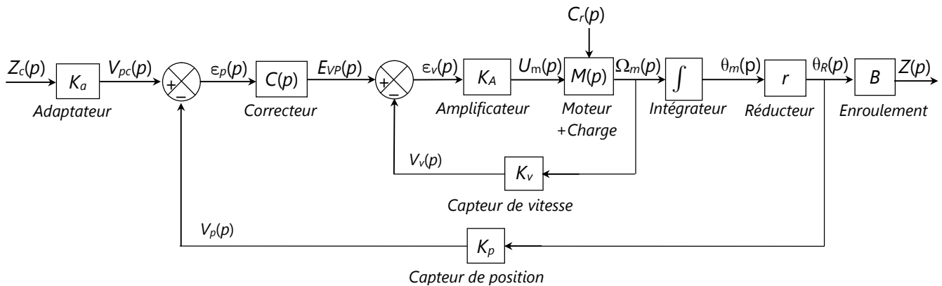
Figure 11 : Asservissement de position avec boucle tachymétrique
