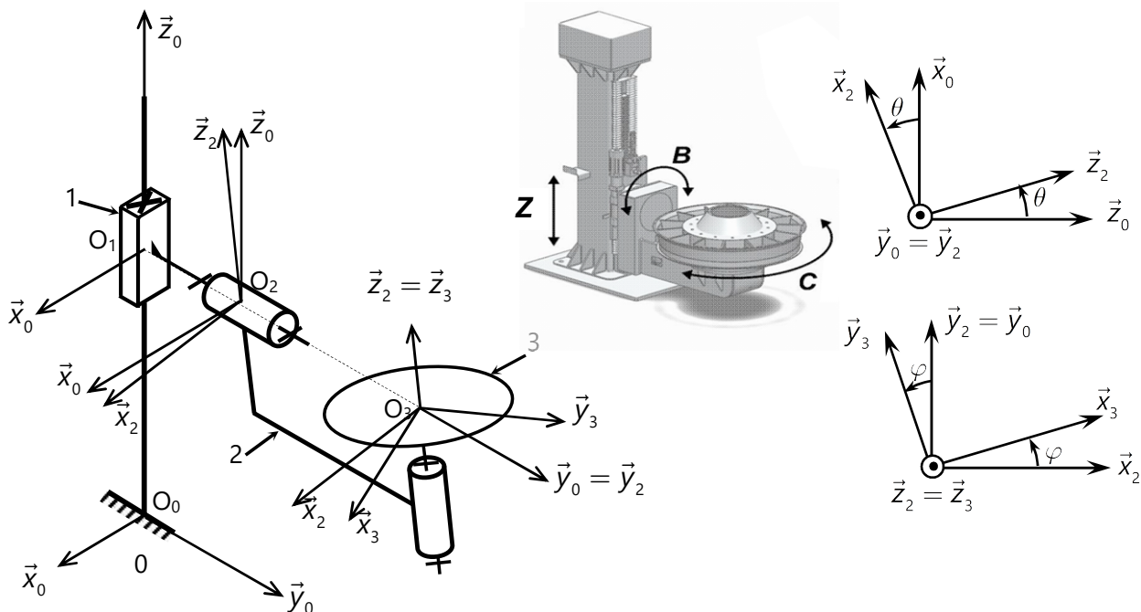
Figure 9 : Schéma cinématique du positionneur
