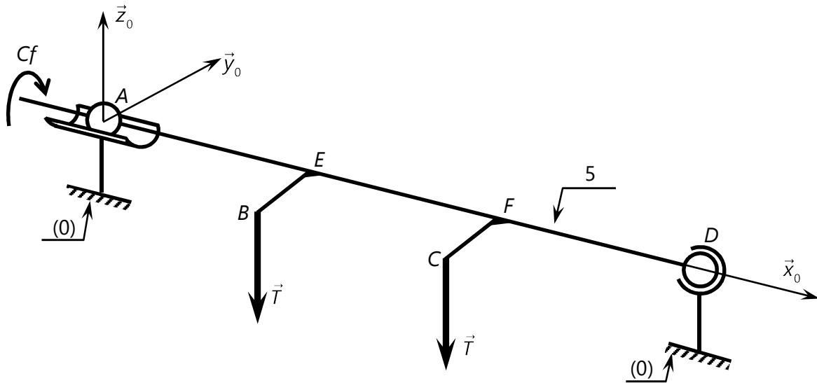
Figure 4 : Modélisation du tambour
