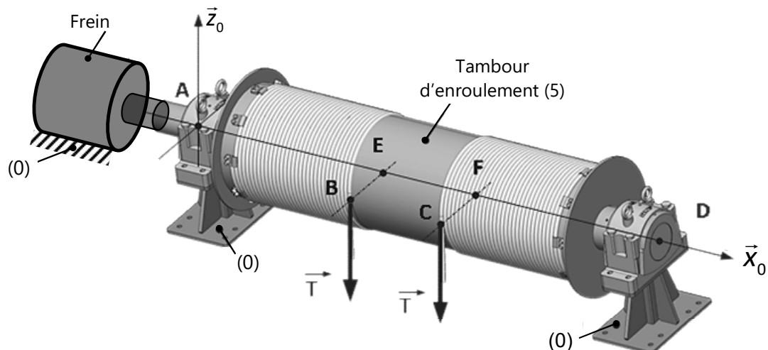
Figure 3b : Enroulement du câble
