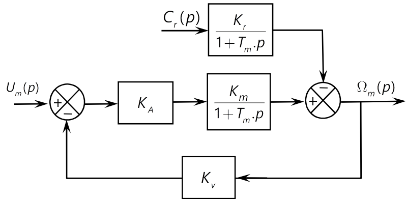
Figure 13 : Schéma bloc du moteur avec chaîne de retour tachymétrique
