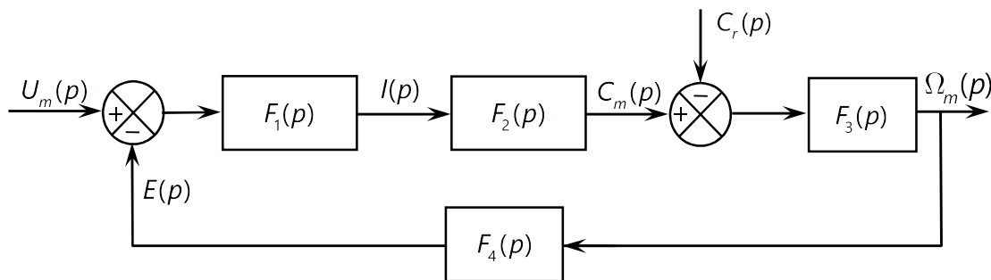
Figure 12 : Schéma-blocs du moteur + charge
