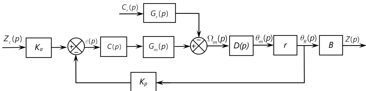
Figure 14 : Schéma-blocs de l'asservissement de position de la montée de la charge
