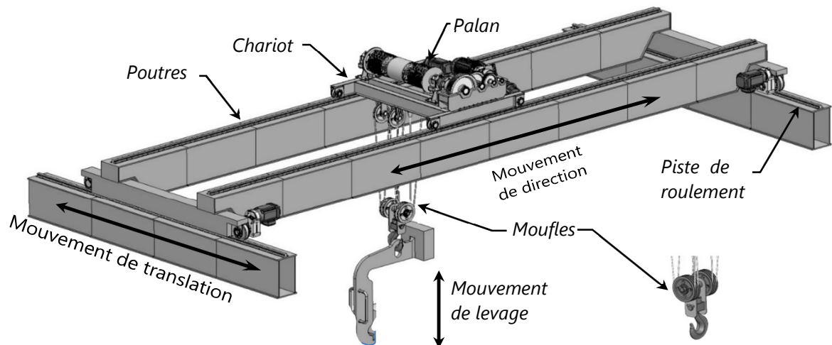
Figure 3a : Système de levage
