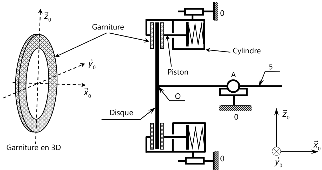
Figure 5 : Système de freinage
