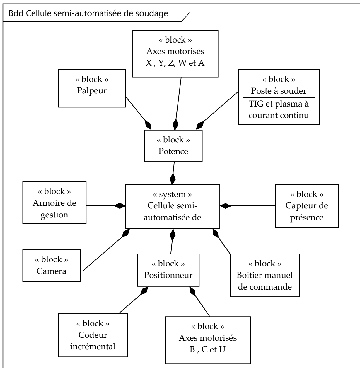
Diagramme de définition des blocs (bdd)
