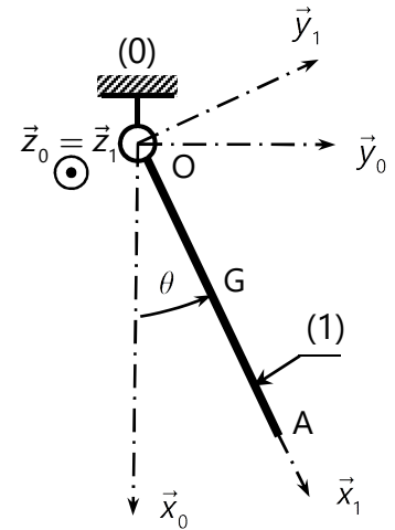
Figure 2 : Bras d'orientation
