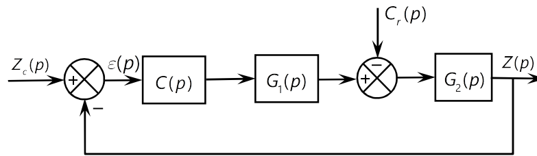
Figure 15 : Schéma-blocs simplifié à retour unitaire
